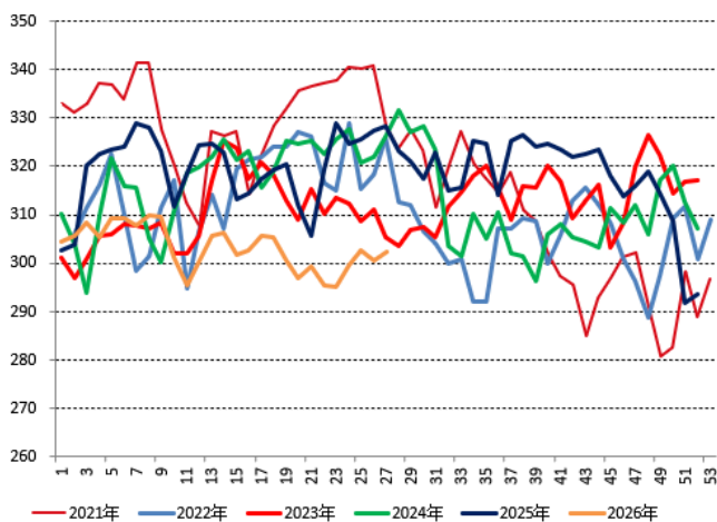
图10 热卷周产量
